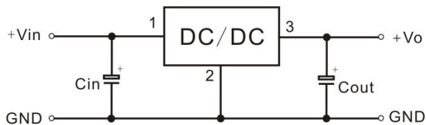
正输出应用电路
